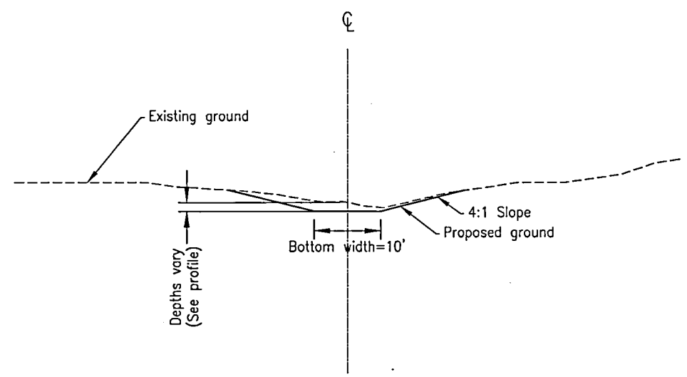
Section A (NTS) Sta. 2+81 to 24+94 Sta. 25+08 to 54+00
