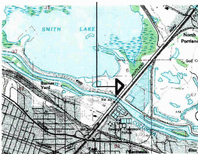
PORTLAND 7.5' QUADRANGLE N.T.S.
