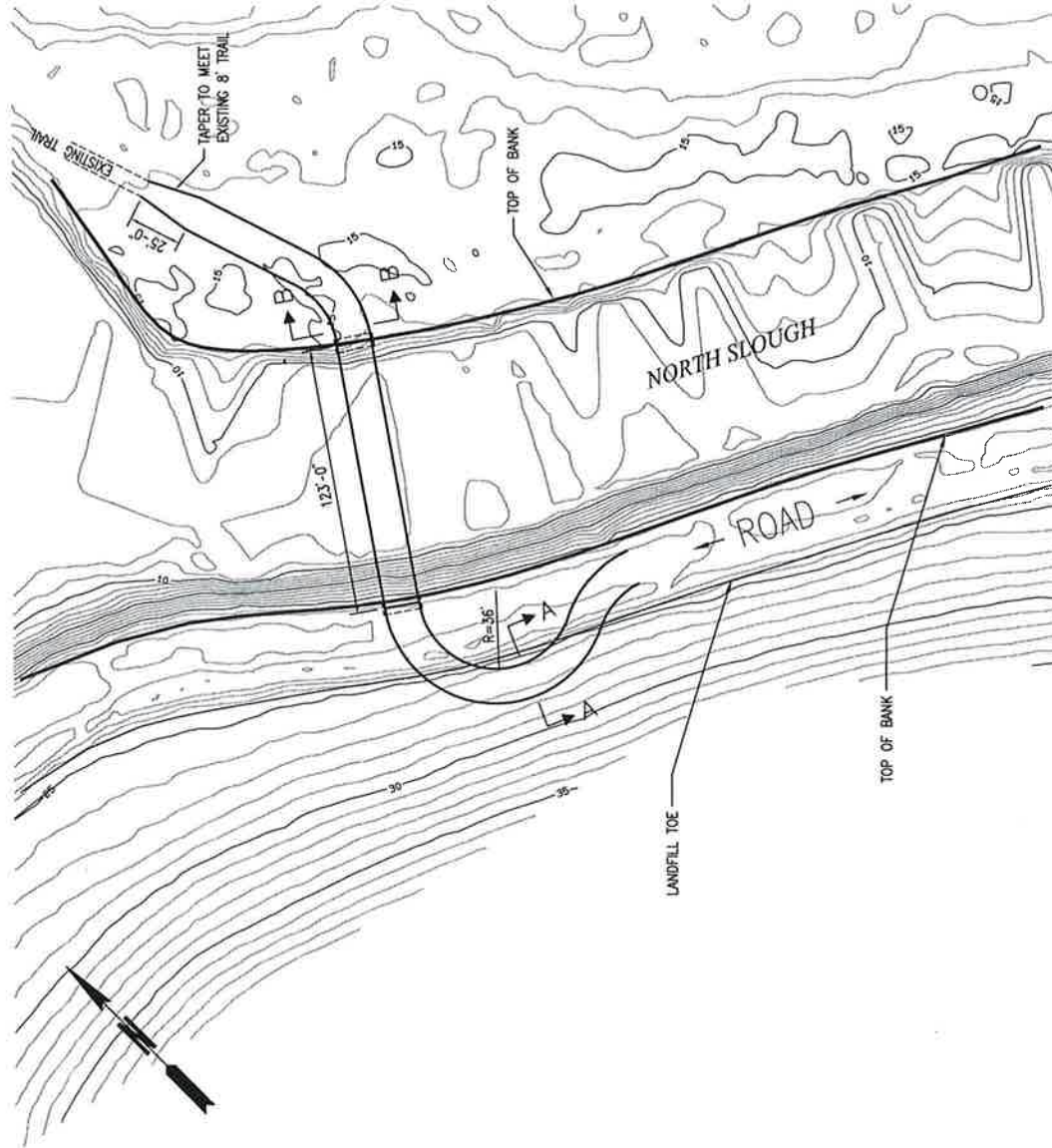
PLAN SCALE: 1" = 60'
